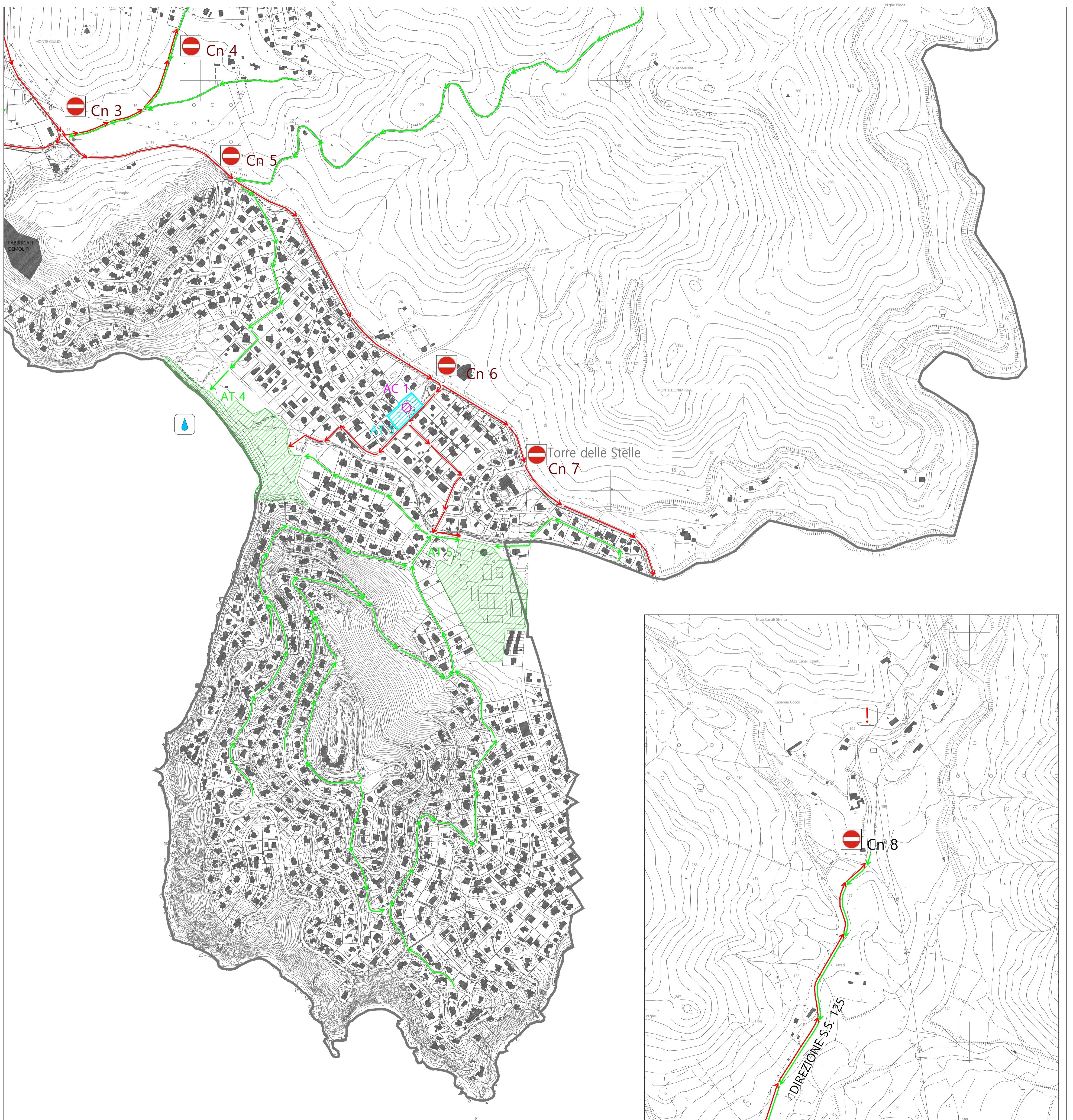
SCENARIO 6 TORRE DELLE STELLE - SCALA 1:5000
